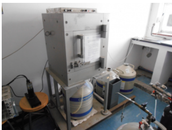
Espectrómetro gamma de Ge Canberra XTRA GX6020.
