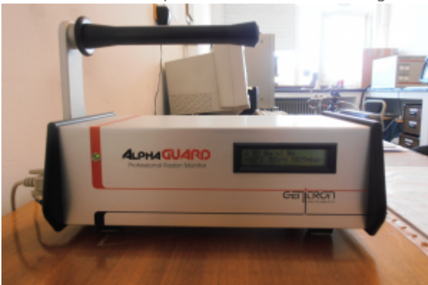
Equipo de medición de radon en continuo Alphaguard PQ 2000PRO
